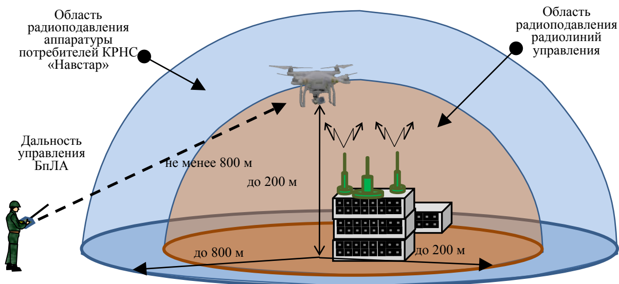
Рис. 13. Вариант применения станции помех РП-377УВМ1Л «Лесочек», при РЭП радиопередачи и аппаратуры потребителя КРНС БПЛА
